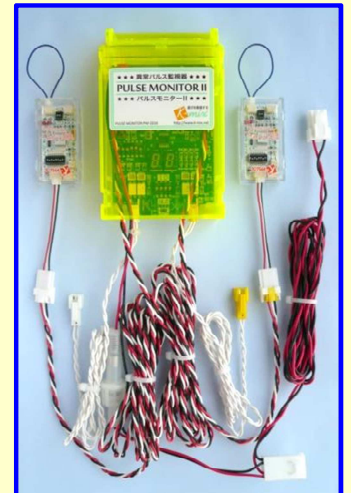
標準仕様(2台管理)
